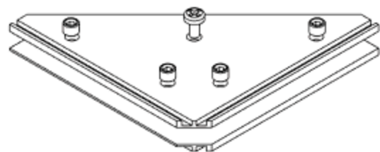
Усилитель угловой для ВВС-30
