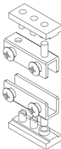
Комплект шарниров для распашной дверки
